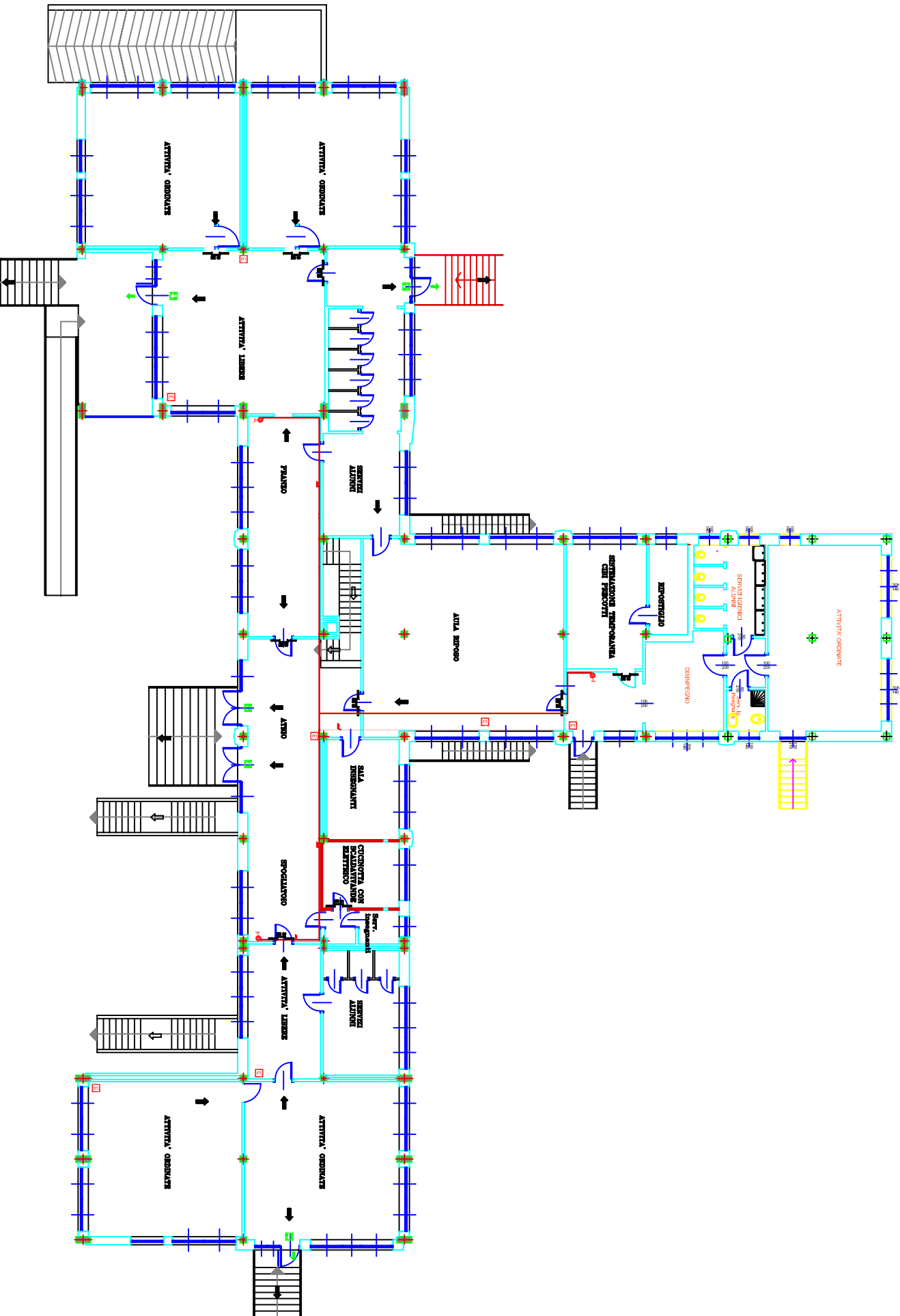
PIANTA PIANO RIALZATO scala 1:250
